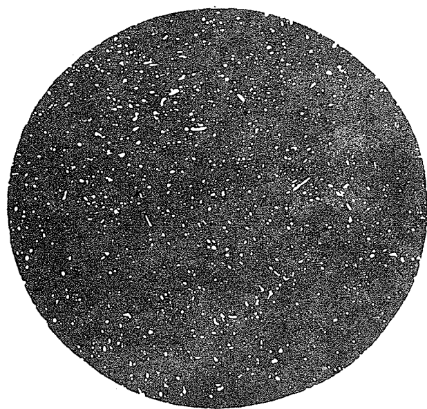
网状碳化物 1级
