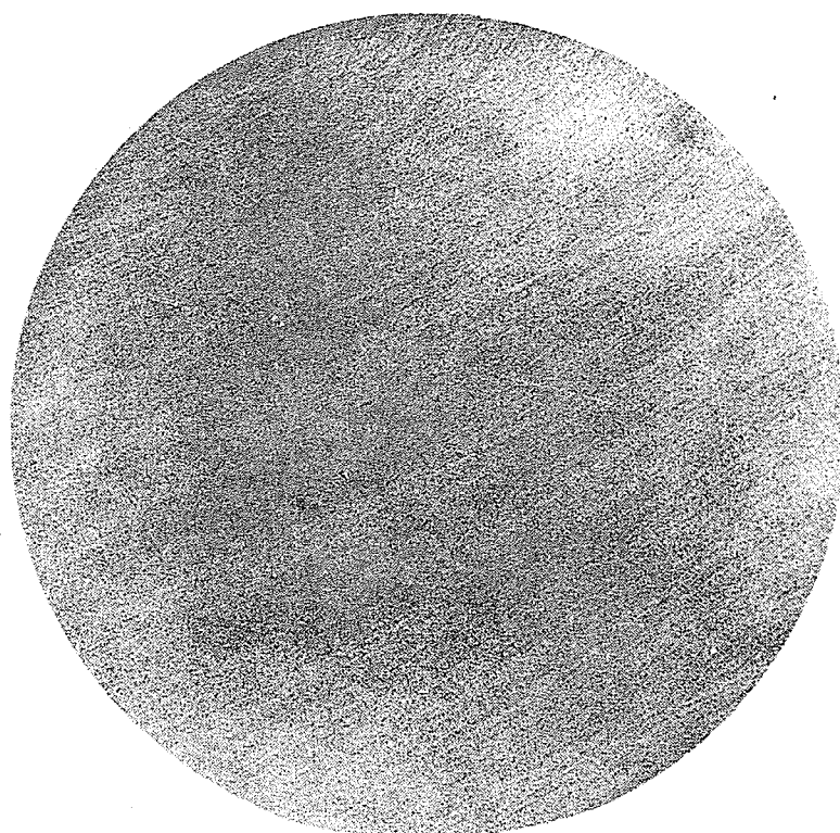
锭型偏析 1级
