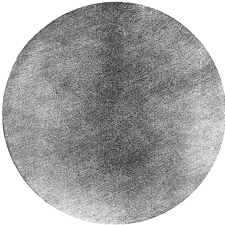
中心疏松 1级
