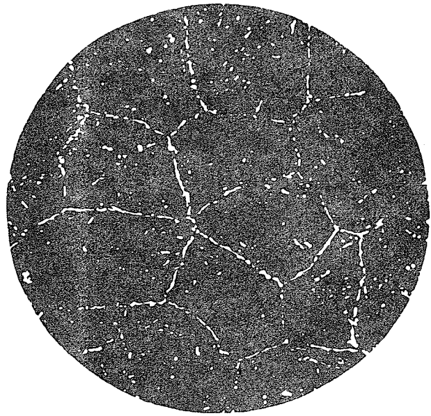
网状碳化物 4级
