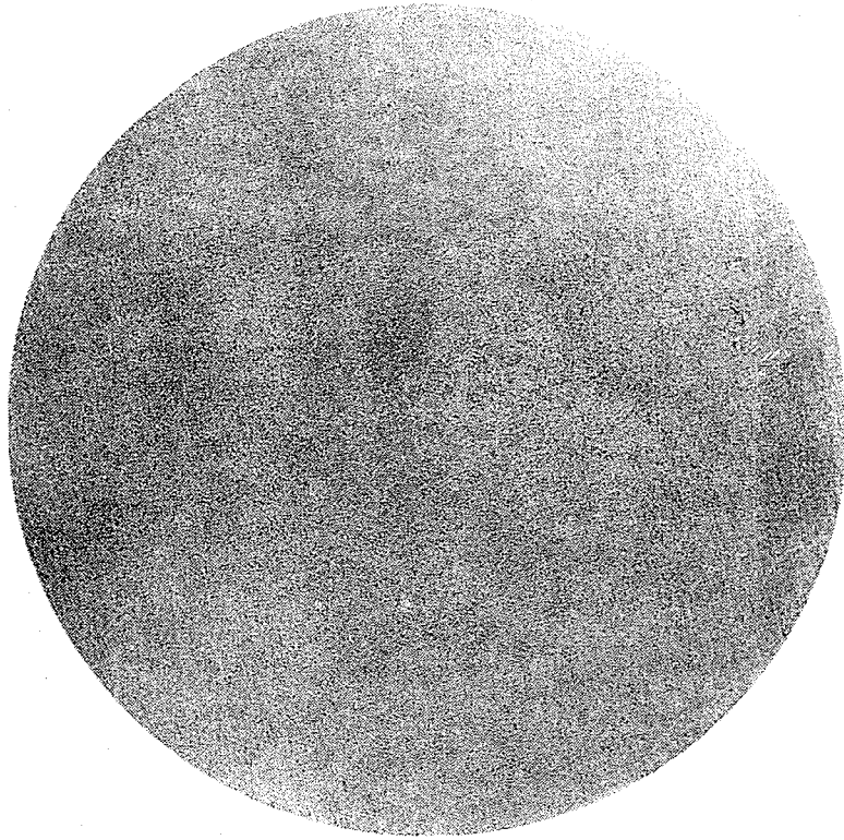
中心疏松 4级
