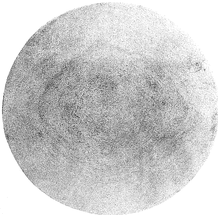
旋型偏析 6级
