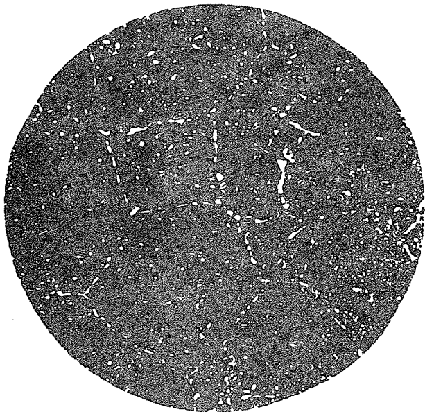
网状碳化物 3级
