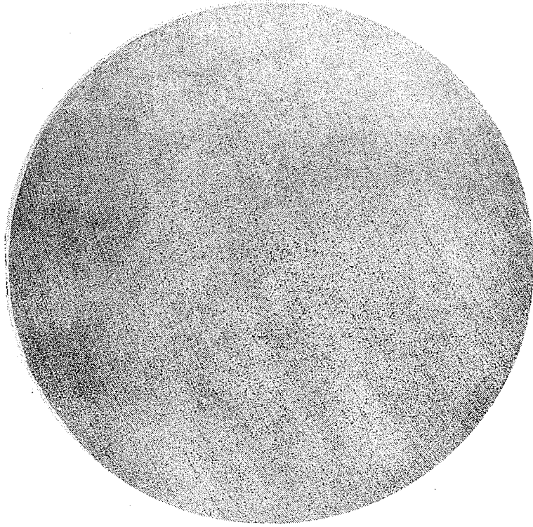
中心疏松 2 级
