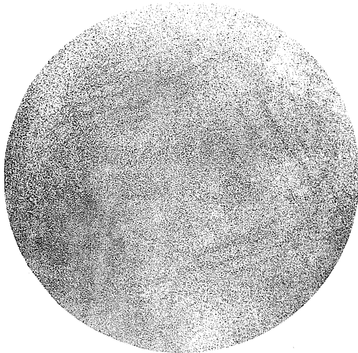
旋型偏析 5 级
