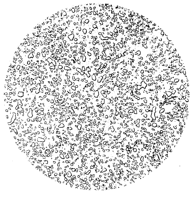
珠光体组织 4级
